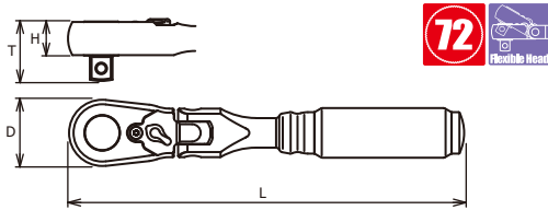
2726Z-160 ⚠ Flexible Ratchet, Reversible Llave de Carraca Flexible, Reversible
